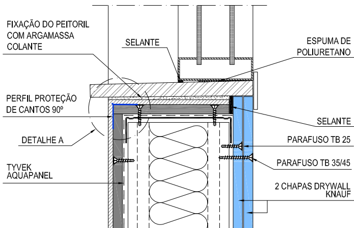
1 PAREDE - JANELA - Corte ESCALA 1:5
