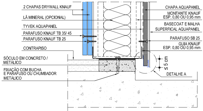
1 PAREDE - MS - Corte ESCALA 1:5
