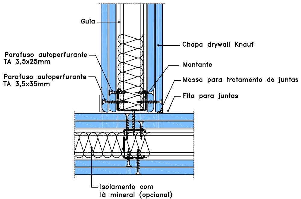
1 DETALHE – ENCONTRO DE PARDE EM T – W112 SEM ESCALA
