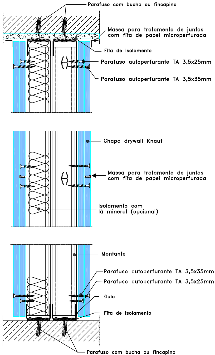
1 CORTE VERTICAL - W115 - EMPS SEM ESCALA
