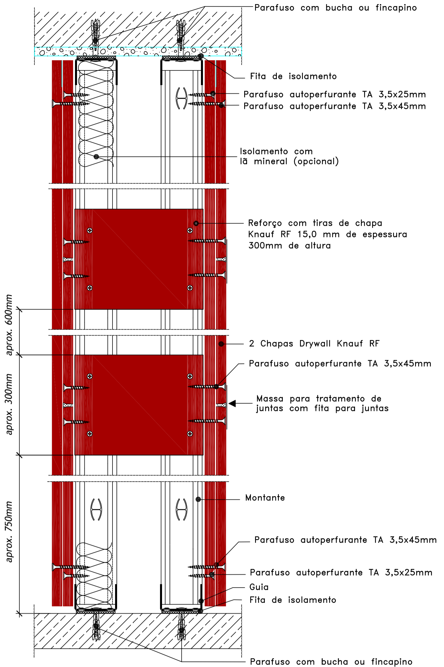
1 CORTE VERTICAL RESISTENTE AO FOGO – RF – W116 SEM ESCALA
