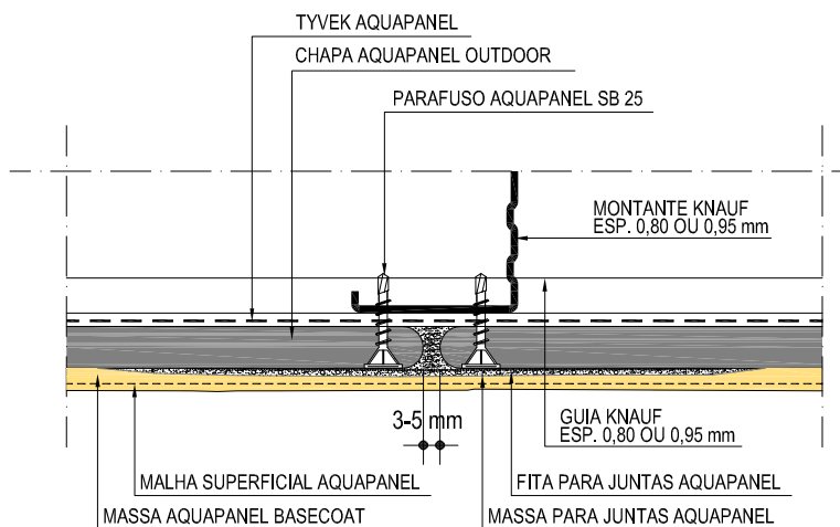
1 PAREDE - MS - Planta Baixa ESCALA 1:5
