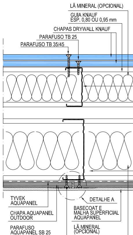
1 PAREDE - MS - Planta Baixa ESCALA 1:5
