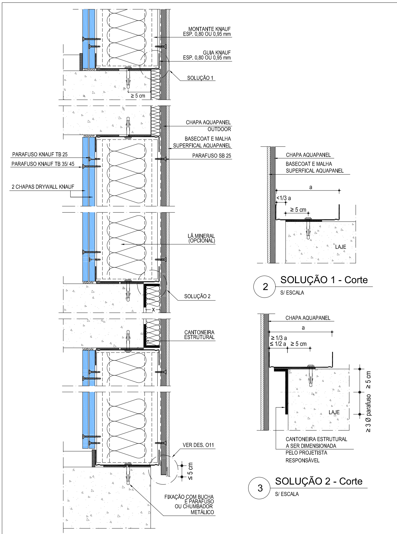
1 PAREDE - MS - Corte ESCALA 1:5
