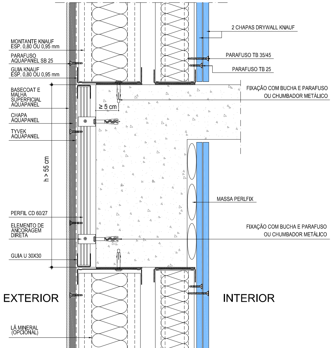
1 PAREDE - ENCONTRO COM VIGA DE BORDA - Corte ESCALA 1:5
