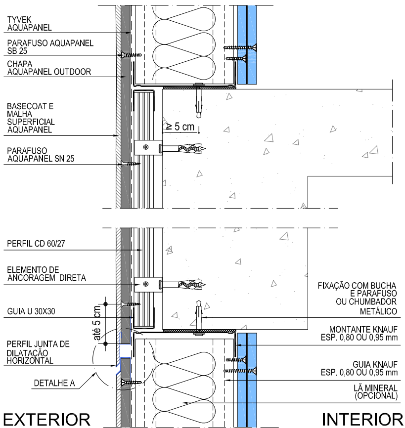
1 PAREDE - JUNTA DE DILATAÇÃO HORIZONTAL - Corte ESCALA 1:5
