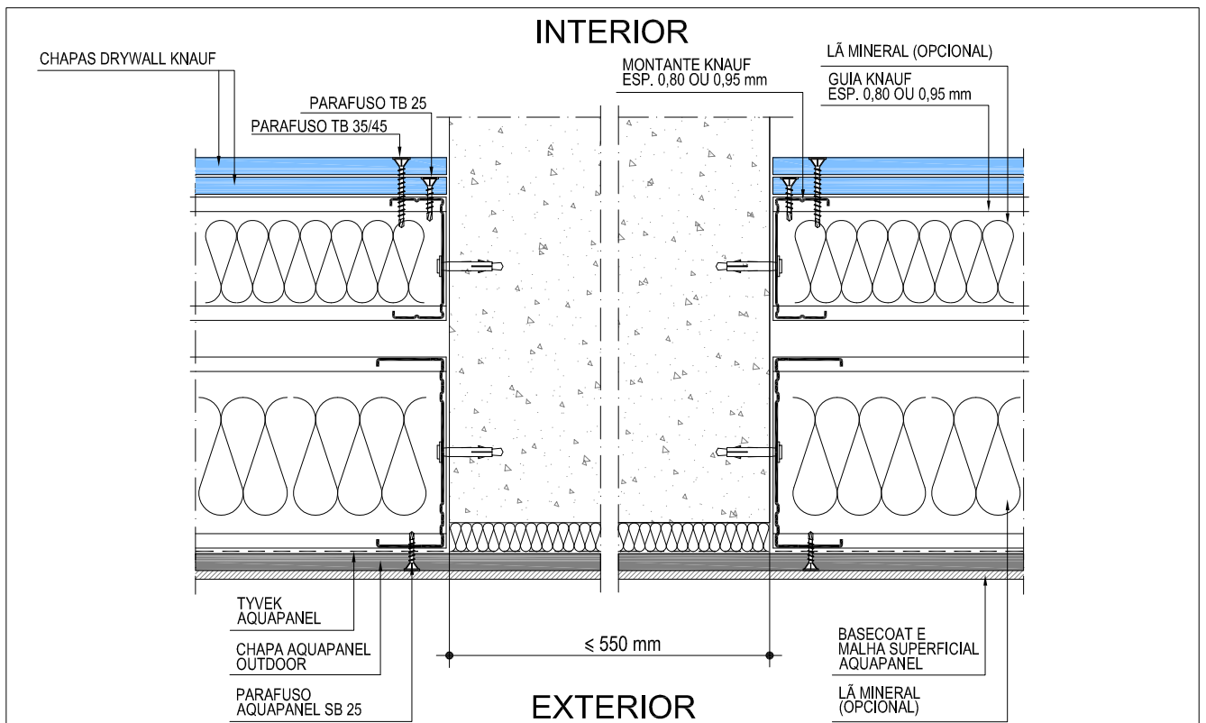
1 PAREDE - ENCONTRO COM PILAR COMPR. < 55cm - Planta Baixa
