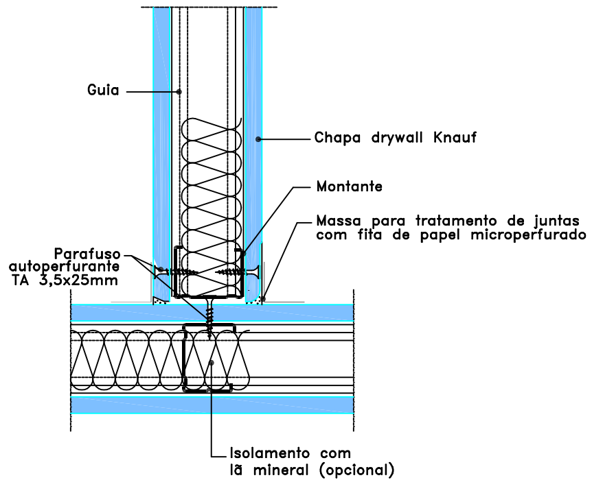
1 DETALHE – ENCONTRO DE PAREDE EM T – W111 SEM ESCALA
