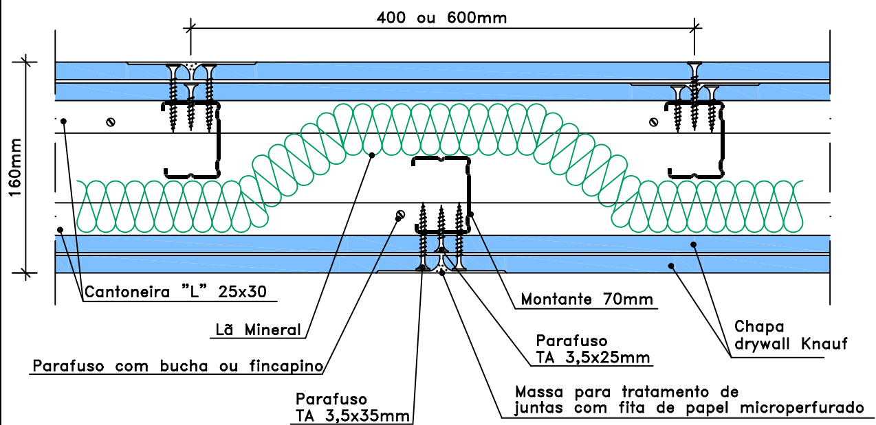
1 CORTE HORIZONTAL – W115 EMAS SEM ESCALA
