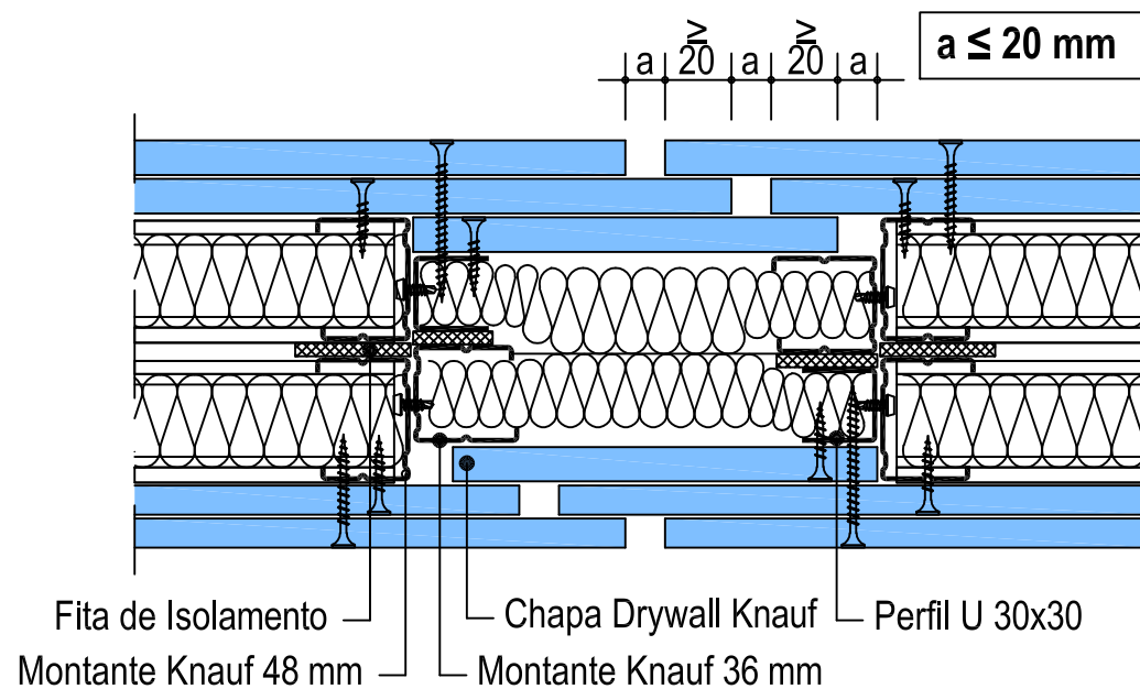
DETALHE - JUNTA DE DILATAÇÃO COM RESISTÊNCIA AO FOGO
