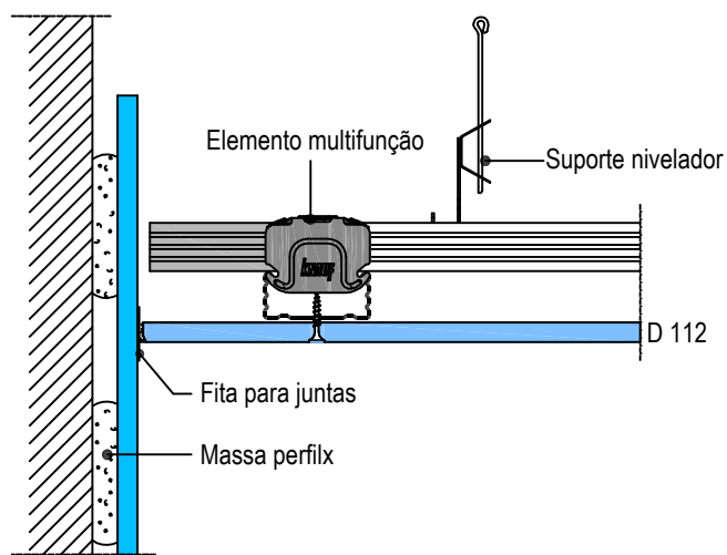
1 ENCONTRO TETO COM REVESTIMENTO W611 SEM ESCALA
