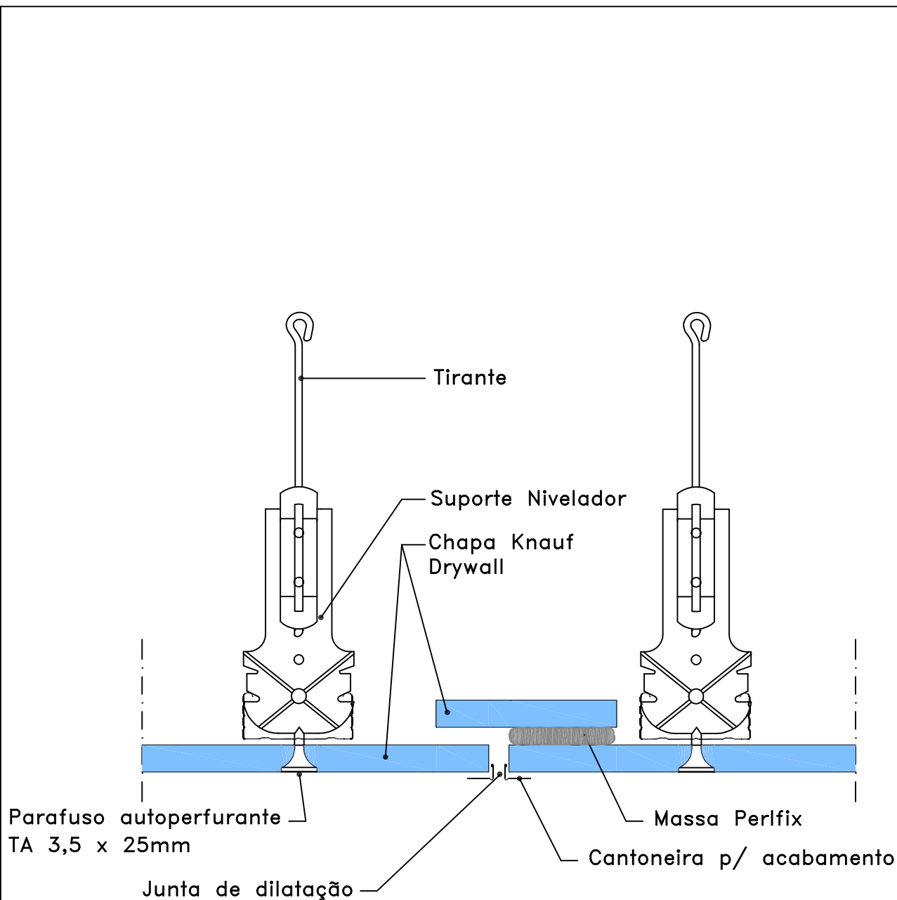
2 DETALHE - JUNTA DE DILATAÇÃO SEM ESCALA
