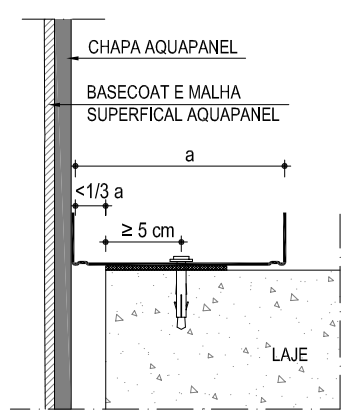
2 SOLUÇÃO 1 - Corte S/ ESCALA
