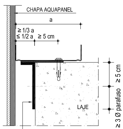
2 SOLUÇÃO 1 - Corte S/ ESCALA
