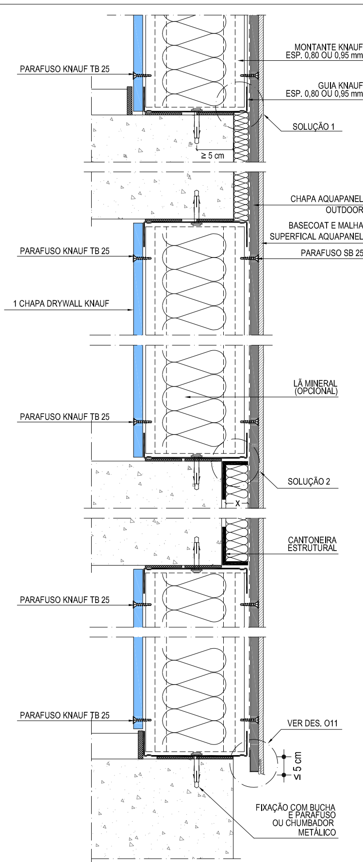
1 PAREDE - MS - Corte ESCALA 1:5
