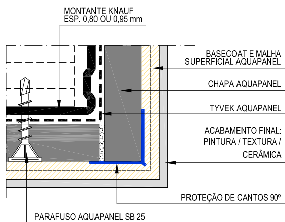
2 DETALHE A - Planta Baixa S/ ESCALA
