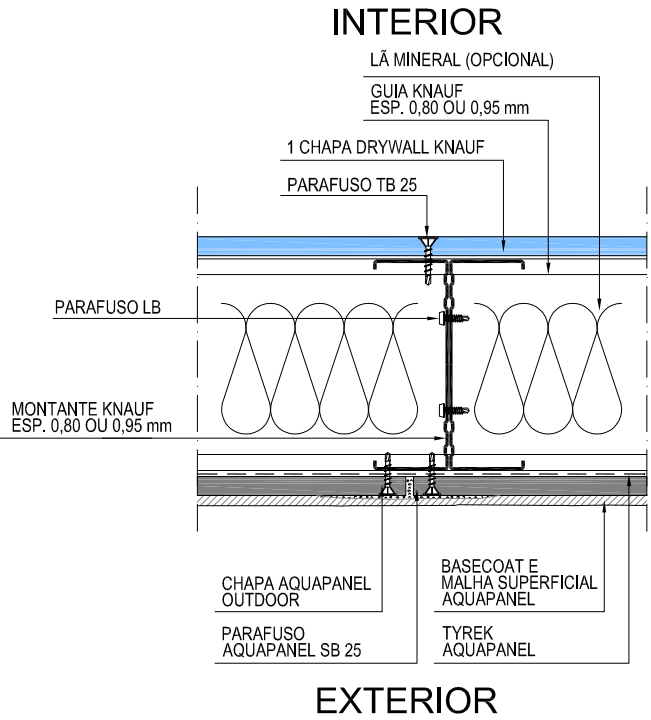
2 PAREDE - MD - Planta Baixa ESCALA 1:5
