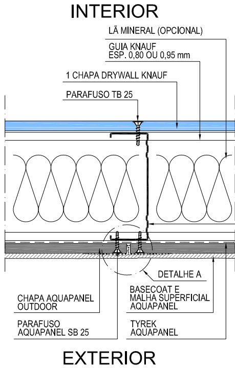
1 PAREDE - MS - Planta Baixa ESCALA 1:5
