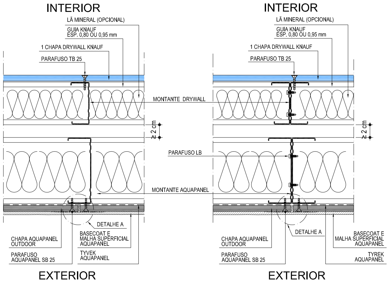
1 PAREDE - MS - Planta Baixa ESCALA 1:5
